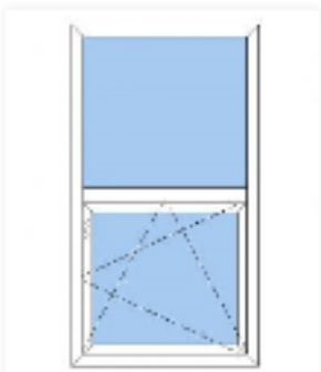
Plast dreje kip en oplukkelig ramme NKPDK-K1-T1
